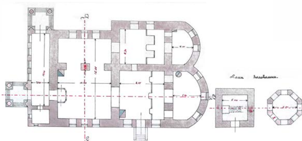
План Казанского храма и колокольни. Чертежи 1926 года
